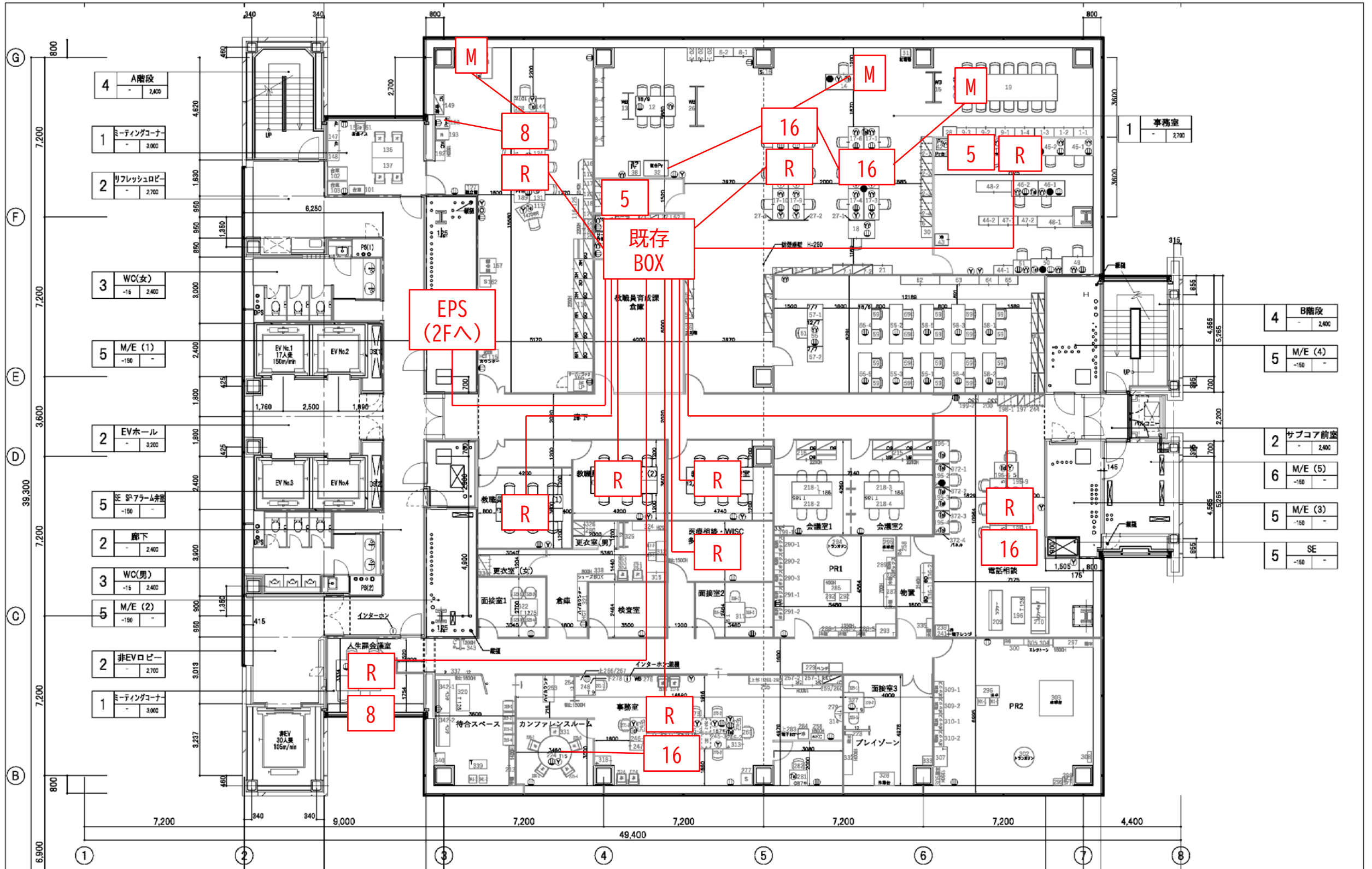
6階YCAN配線図 (ケーブル色：白) R：床下ローゼット M：マグネット付きモジュージャック 数字：HUBポート数
