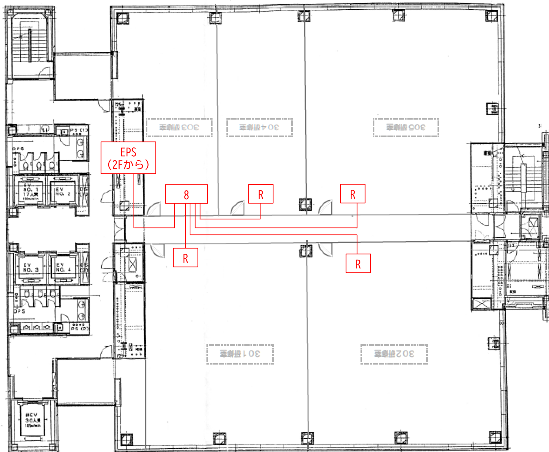
3階予備ネットワーク配線図 (ケーブル色：白) R：床下ローゼット (鍵付き) 数字：HUBポート数
