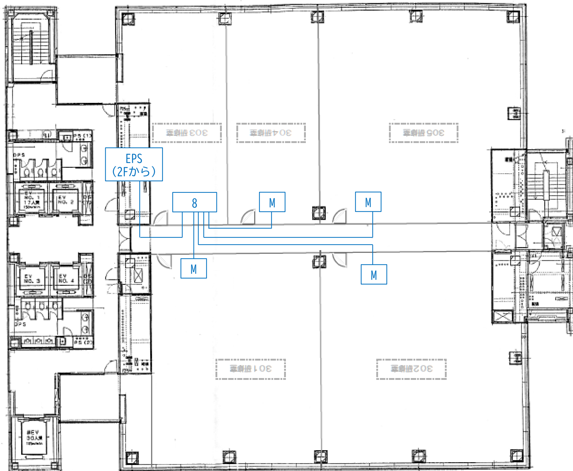
3階Y・Y NET配線図 (ケーブル色：濃い青) M：壁付けモジュージャック 数字：HUBポート数
