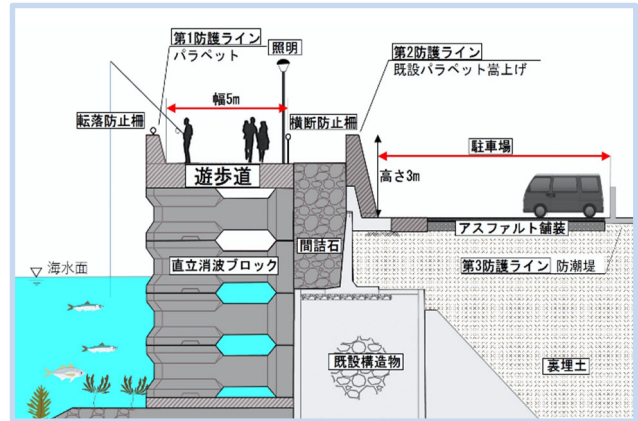
▲断面図（護岸の背後は駐車場として整備）
