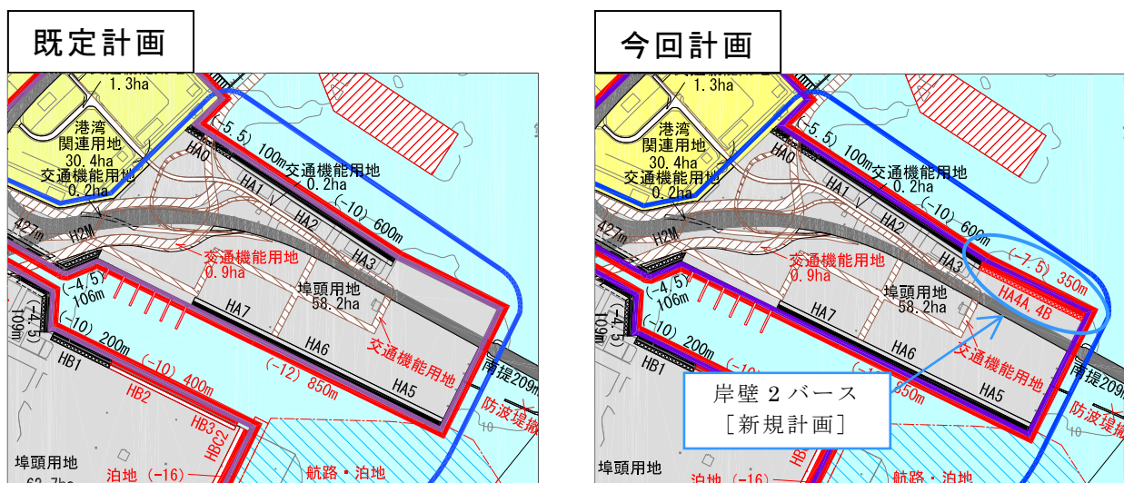
図2-2-1 公共埠頭計画(本牧ふ頭地区)の位置
