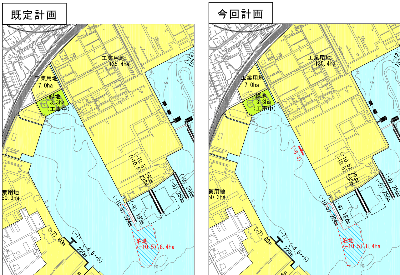
図 3-2-1 専用埠頭計画（磯子地区）の位置
