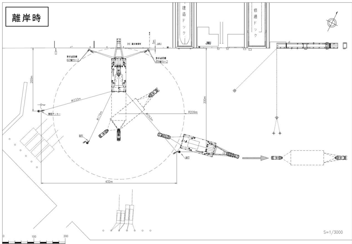
図3-2-2 操船図
