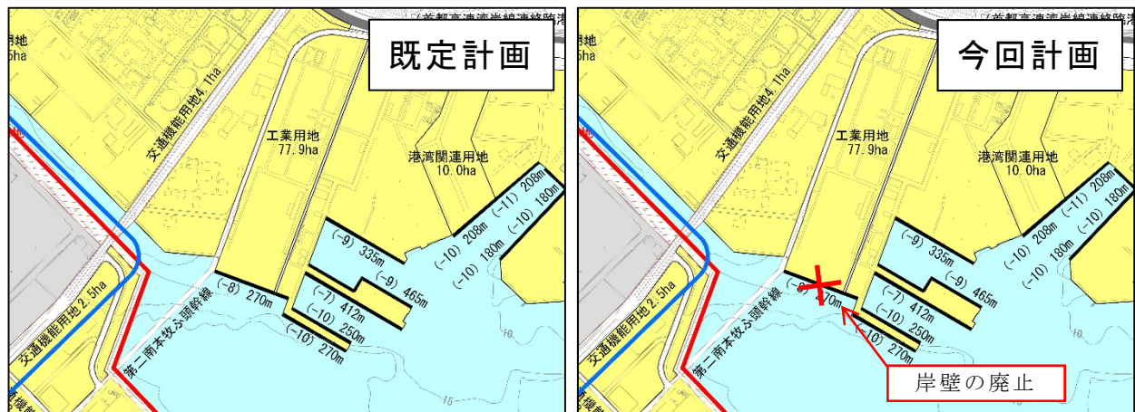
図2-2-1 専用埠頭計画（本牧地区）の位置
