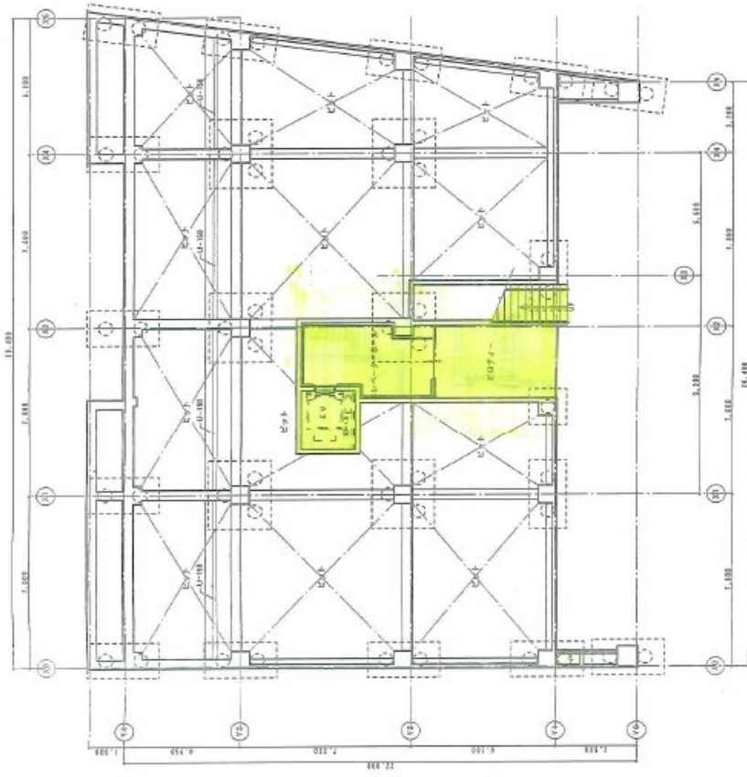
地階平面図 縮尺1/200
