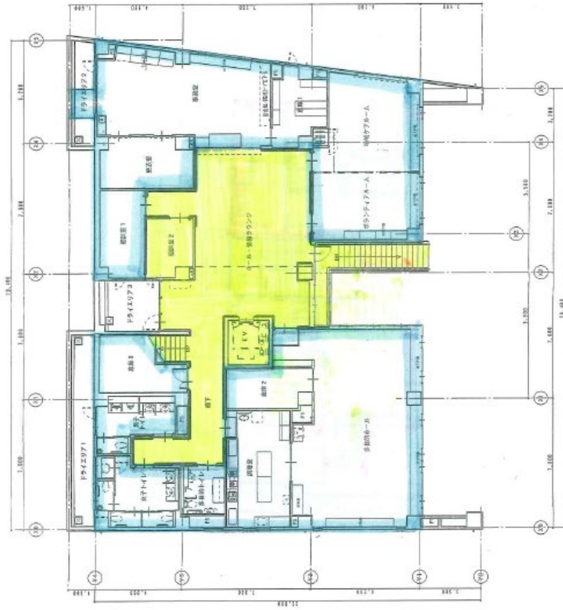
1階平面図 縮尺1/200
