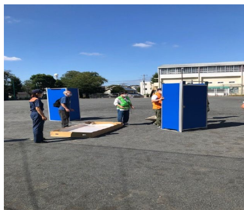
下水道直結式トイレの組立
