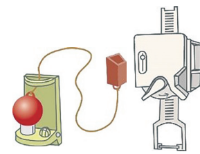
▲安装在配电盘上的简易型号感震闸(示例)
