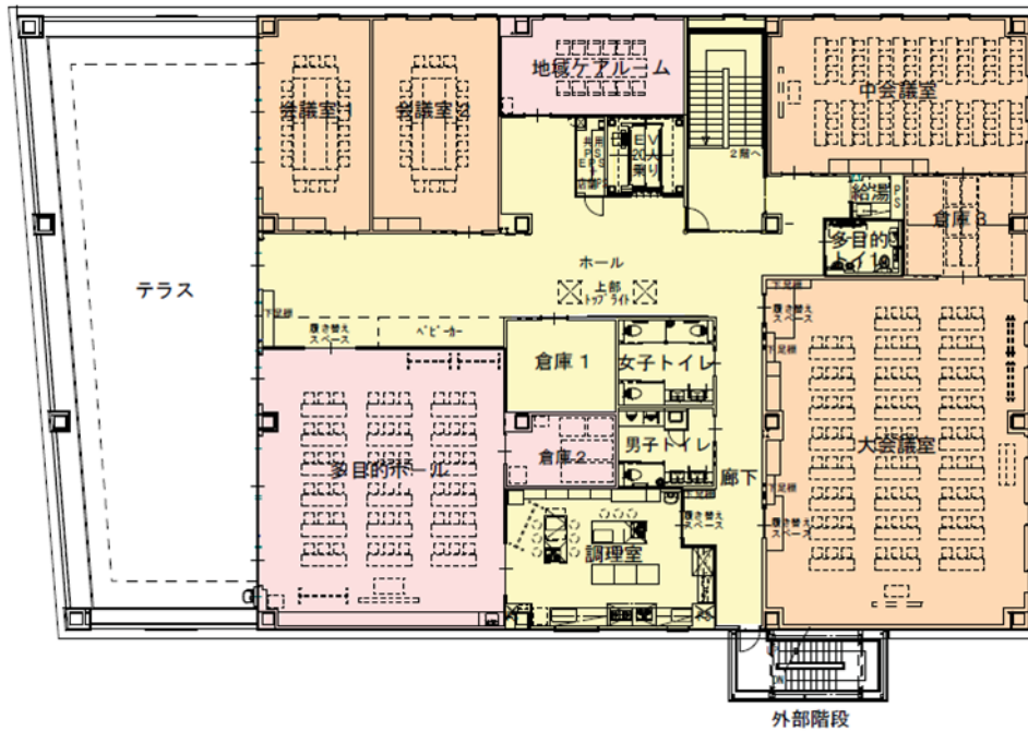
3 F 平面図
