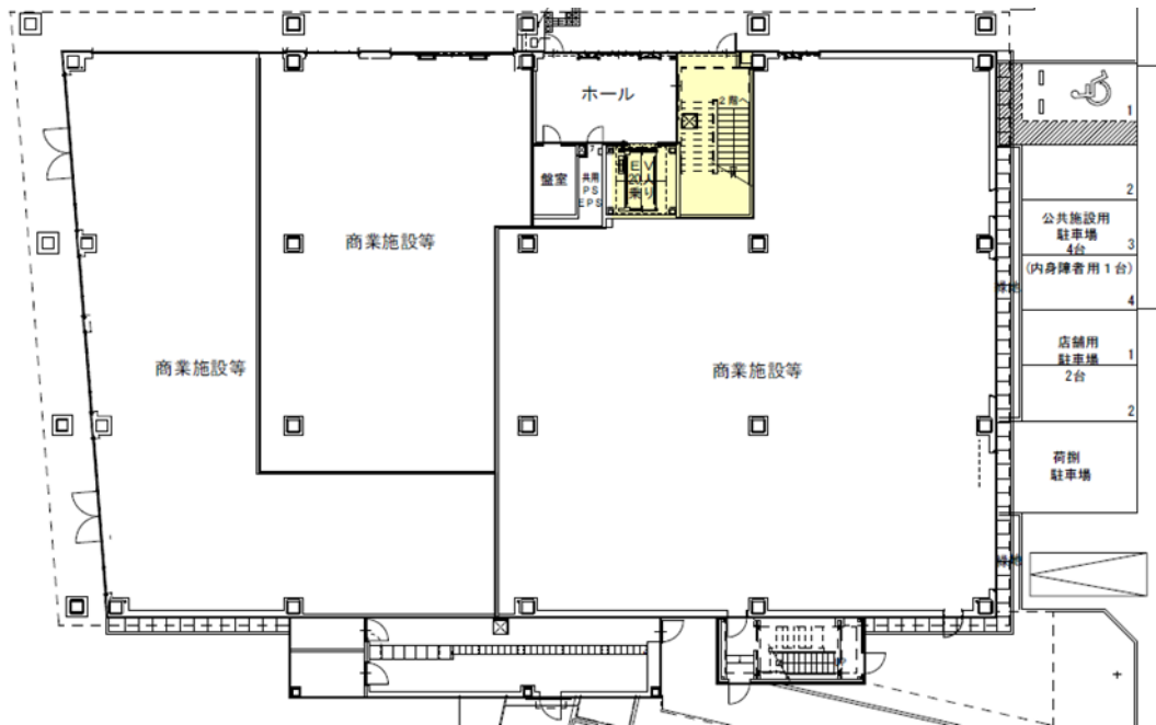
1 F 平面図
