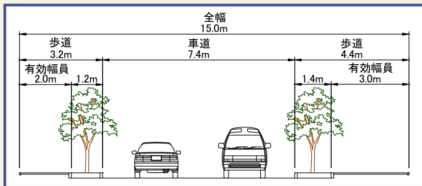
瀬谷区役所前通り 整備後の道路断面図
