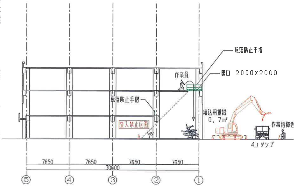
A-A断面図
