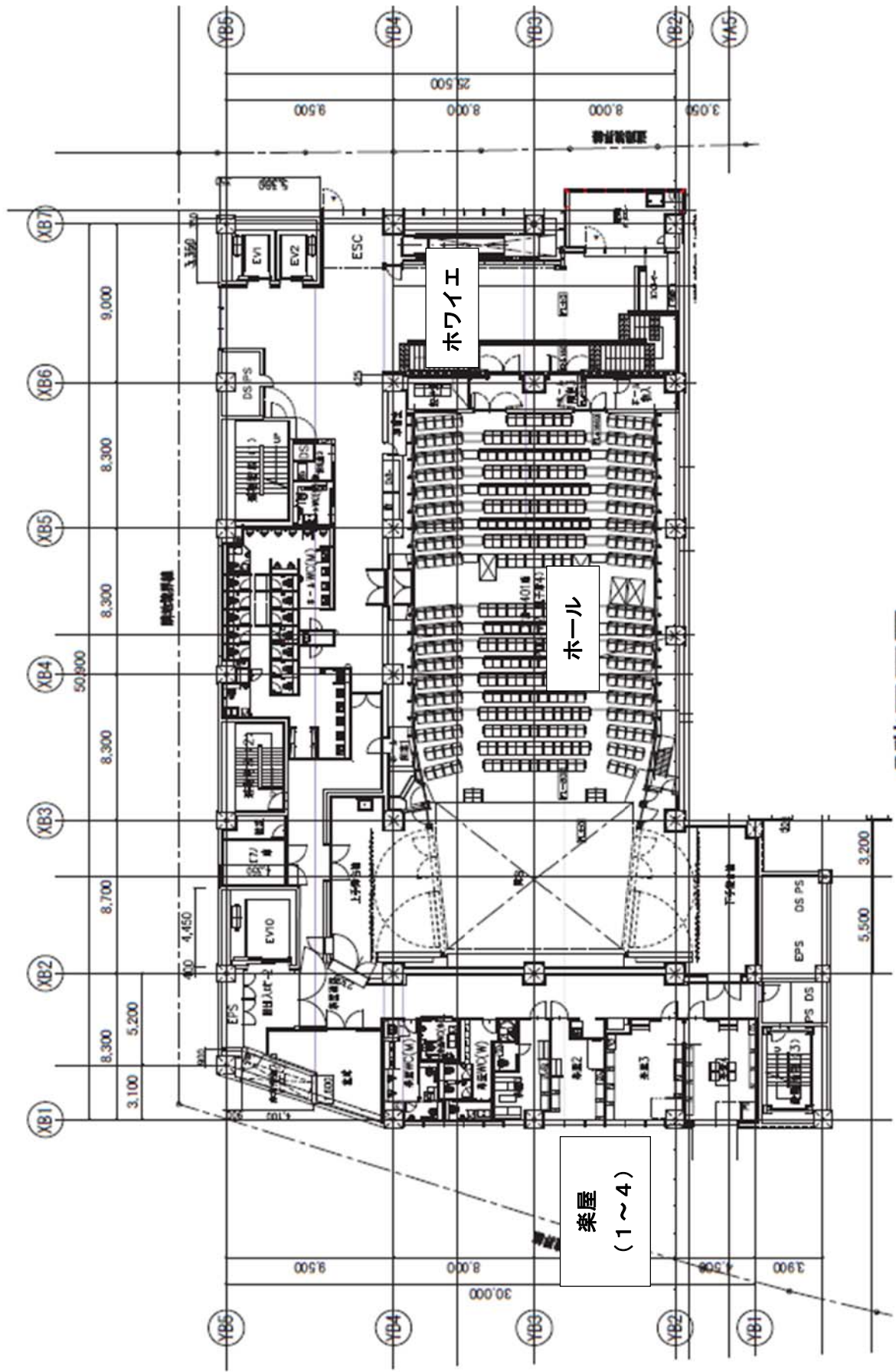
5階平面図
