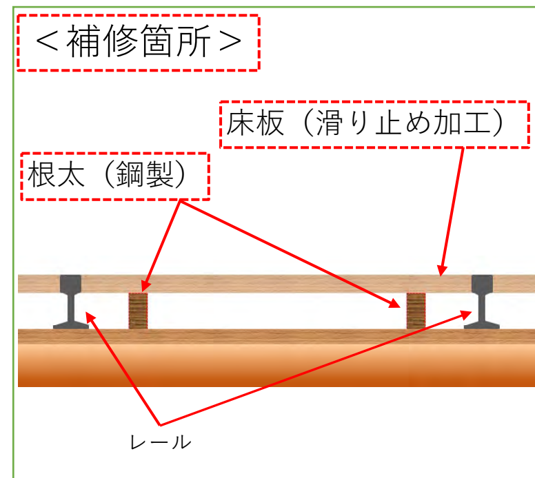
施工断面イメージ
